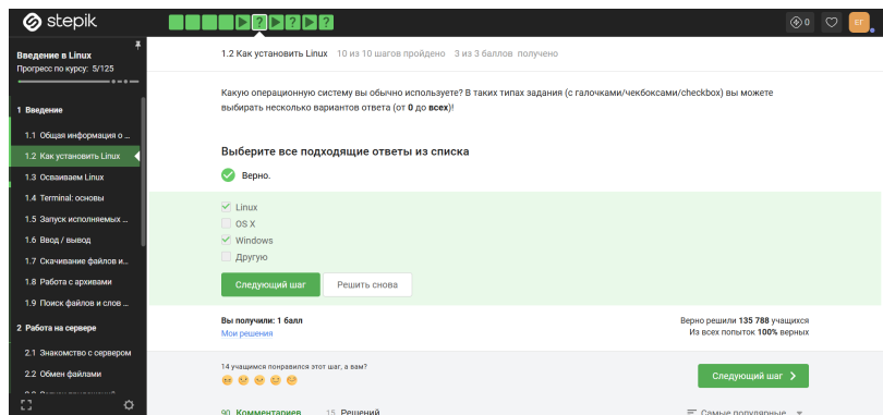
Рисунок 2.3: ОС
